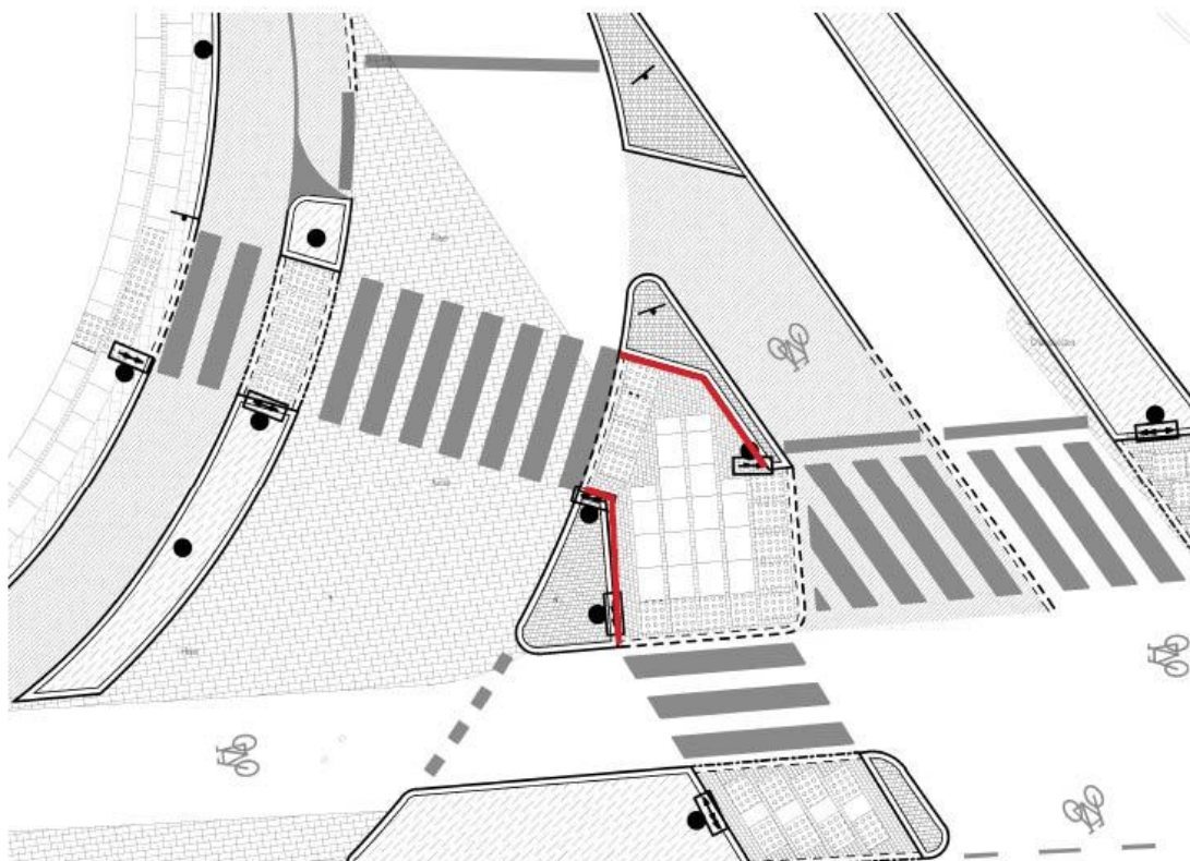
Figur 7. Ny cykel ø og fodgængerhelle. Rød markering visende kantstenslysning.
