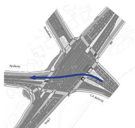
Figur 6. Blå pil visende bilisternes mere rette krydsning af Ring 2 efter ombygning.
