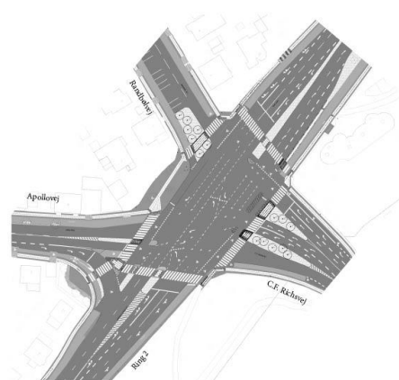
Figur 2. Situationsplan af 5-benet krydsløsning. Kort: Via Trafik.
