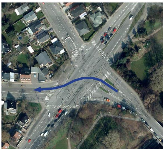
Figur 5. Blå pil visende bilisternes knækkede krydsning af Ring 2 før ombygning.
