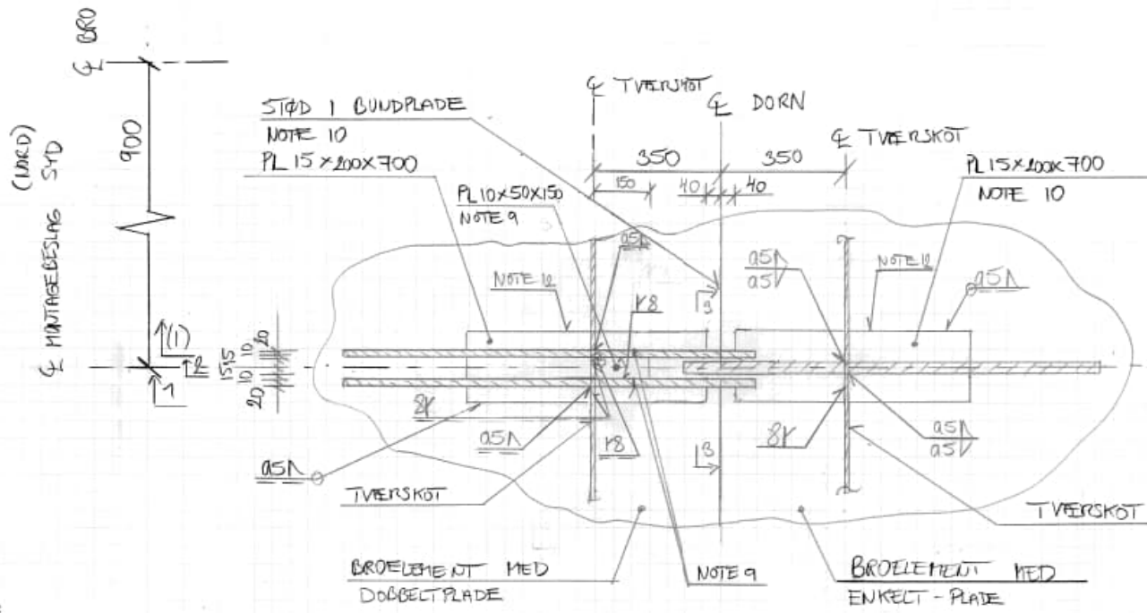
Snit A-A 1:10 Se tegning 21 og P.P. for svejseanordninger mellem tværskøt og broelement.
