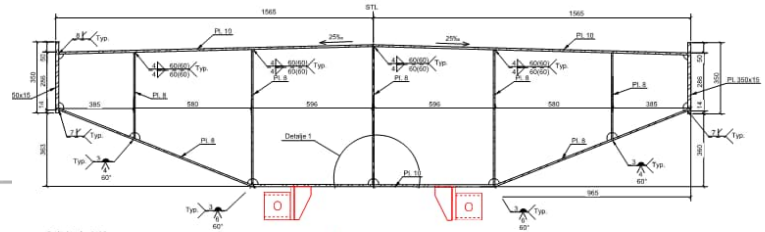
Snit A-A 1:10 Se tegning 21 og P.P. for svejseanordninger mellem tværskøt og broelement.
